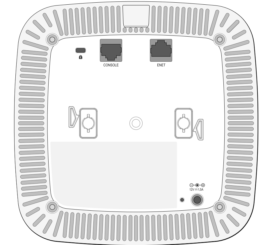
图 3 W-AP110 系列后视图
