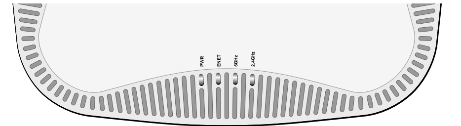
图 1 W-AP110 系列 LED
