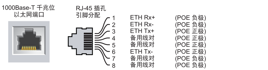
图 5 千兆位以太网端口引脚分配
